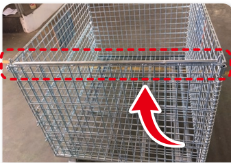
補強① 上部フレーム補強
