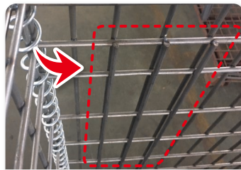
補強② 側面パネル補強
