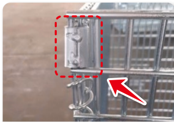
補強③ カシメ溶接補強
